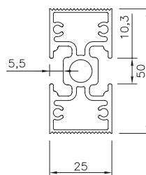
Misure profilo InUno
