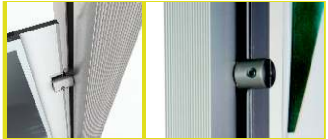
Morsetto in alluminio anodizzato per fissaggio diretto
