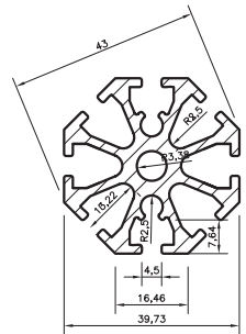
Sezione montante
